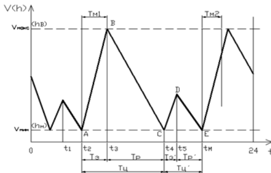
Рисунок 2 - Організація роботи водовідливної установки при керуванні по трьох точках, де T_{ц} і T_{ц}' – тривалість відповідно повного і передпікового циклів роботи водовідливної установки; T_{з} і T_{з}' – тривалість відповідно заповнення водозбірника в повному і передпіковому циклах; T_{р} і T_{р}' – час продуктивної роботи насосного агрегату відповідно в повному і передпіковому циклах
