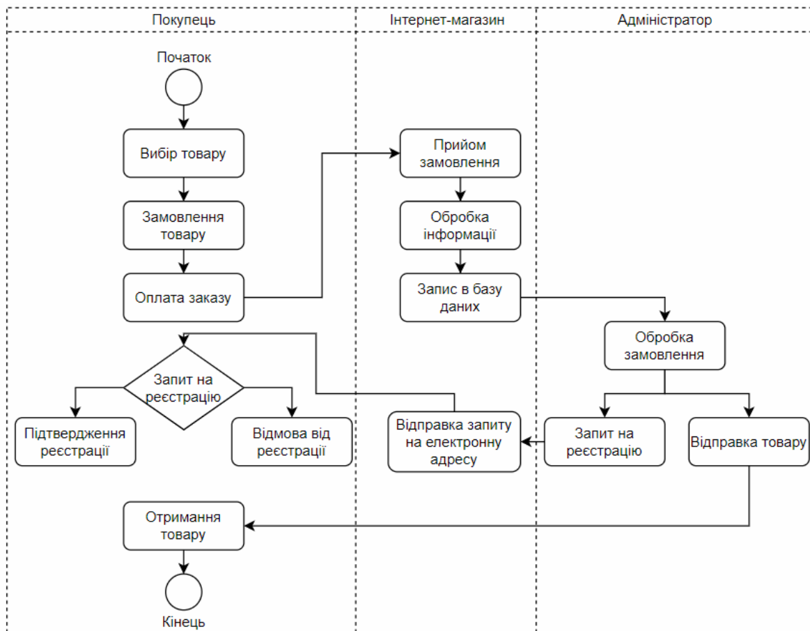
Рисунок 3 Диаграма діяльності
