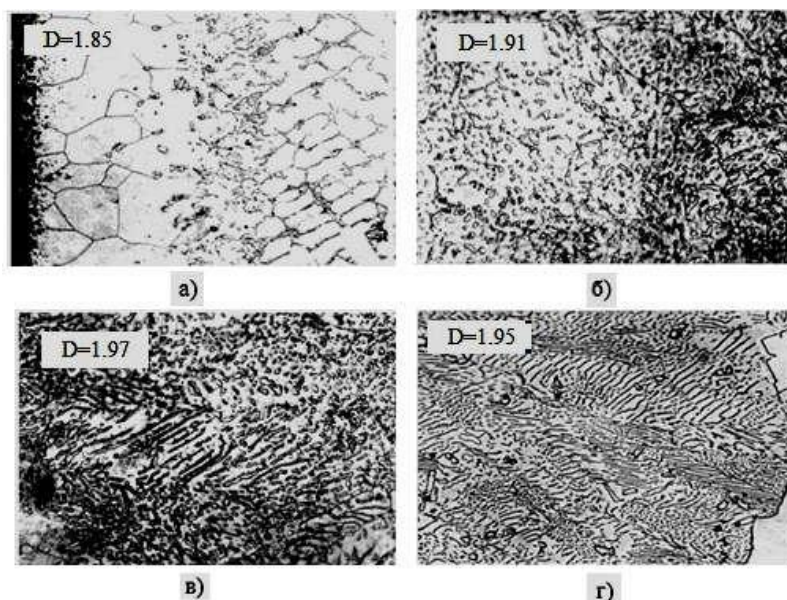
Рисунок 4 - Сталь Р6М5. Процес формування композитної структури швидкоріжучої сталі Р6М5: а) знеуглецьований поверхневий шар; б) науглецювання 30 хвилин; в) науглецювання 1 година; г) науглецювання 2 години - кінцева структура
