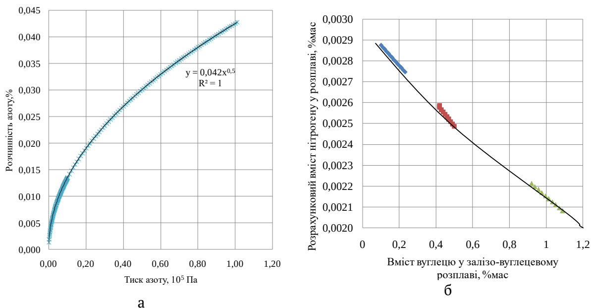
Рисунок 1 – Залежність кількості розчиненого нітрогену у розплаві від початкових умов: а - від тиску газоподібного нітрогену над розплавом; б - від вмісту вуглецю у трьох типах залізовуглецевих розплавів (відповідно до обраного у розрахунку хімічного складу)
