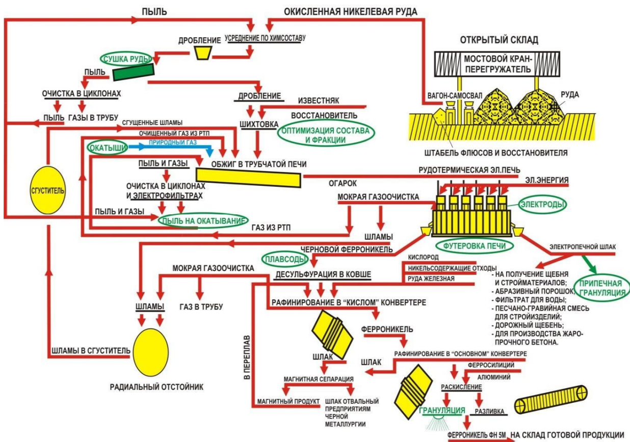
Рисунок 1 – Технологическая схема производства ферроникеля на ООО «ПФК»
