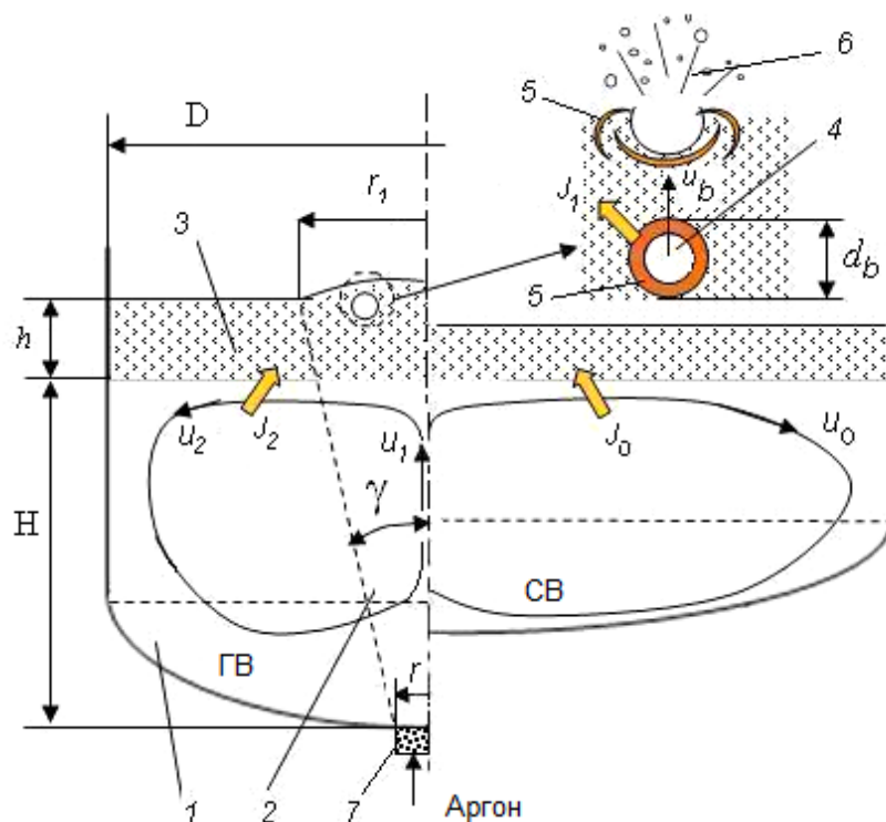
Рисунок 1 – Схема процесу десульфурації в ДСП зі стандартною (СВ) і «глибокою» (ГВ) ванною з пневматичним перемішуванням:
