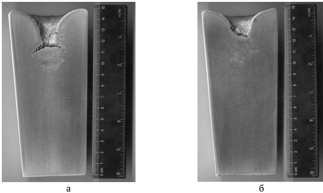
Рисунок 6 - Макроструктура виливків, що отримані в кокіль з додаванням 0,2 мас. % SiC (а) та 0,3 мас.% SiC (б)
